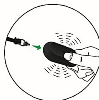
Dimensiones: 7.15L x 3.15A x 1.30 (cm.) Peso: 20 gr Materiales: Plástico ABS | Aluminio Volumen: 120 dB Baterías: CR1632 3V
