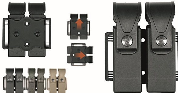
8DMH01 PORTA CARGADOR UNIVERSAL DOBLE PISTOL MAGAZINE CASE PORTE CHARGEUR DOUBLE En polímero, con pasador de doble posición horizontal/vertical Tapa regulable y extraíble que posibilita que quede abierto.
